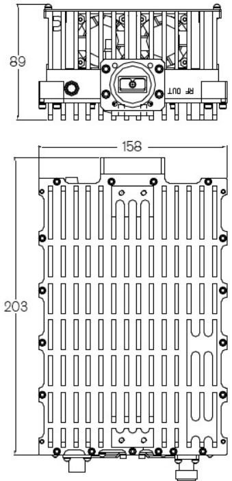
Рисунок 1 – BUC с питанием от сети постоянного тока
